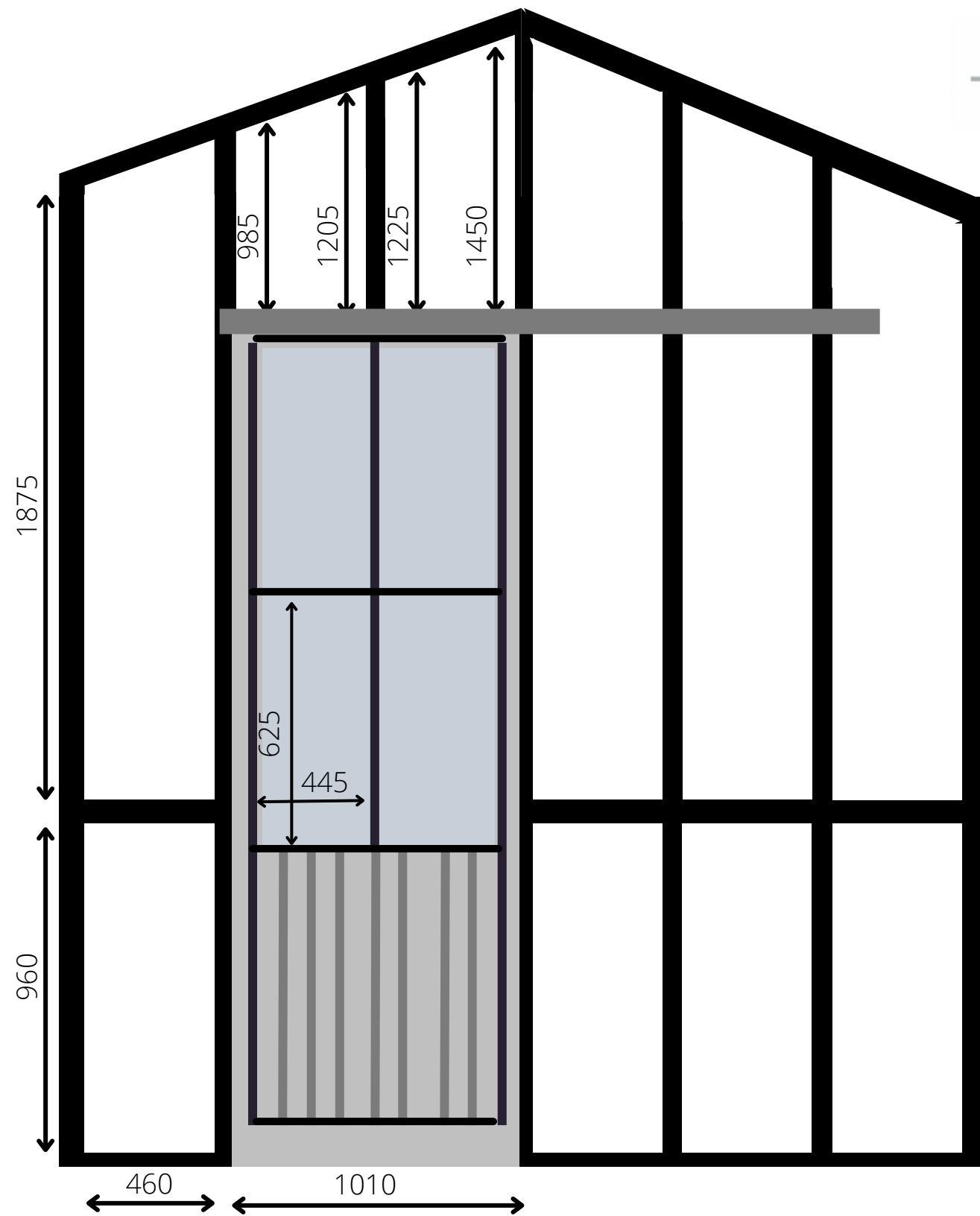
AFMETINGEN VOORGEVEL MET DEUR
