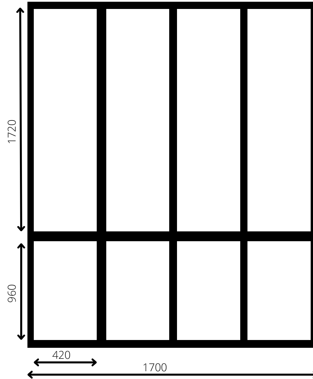
AFMETINGEN ZIJGEVEL
