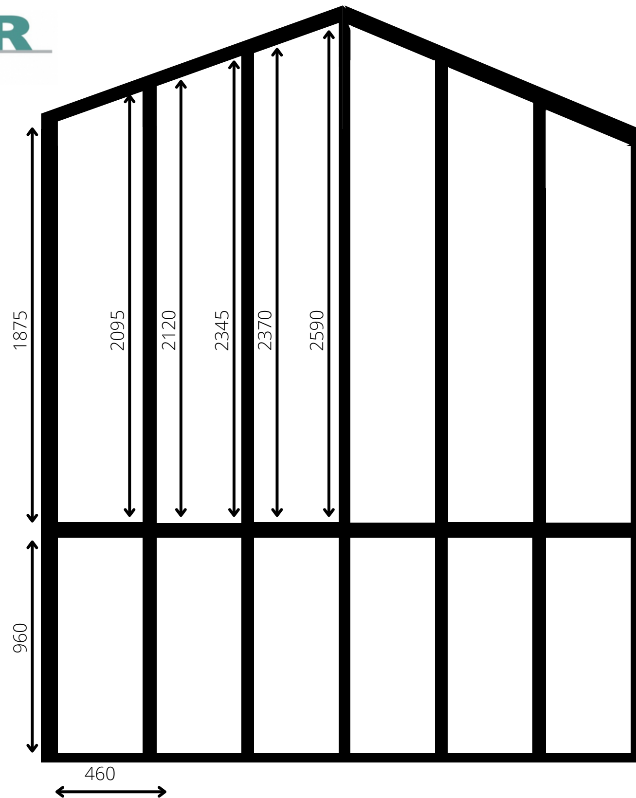
AFMETINGEN ACHTERGEVEL
