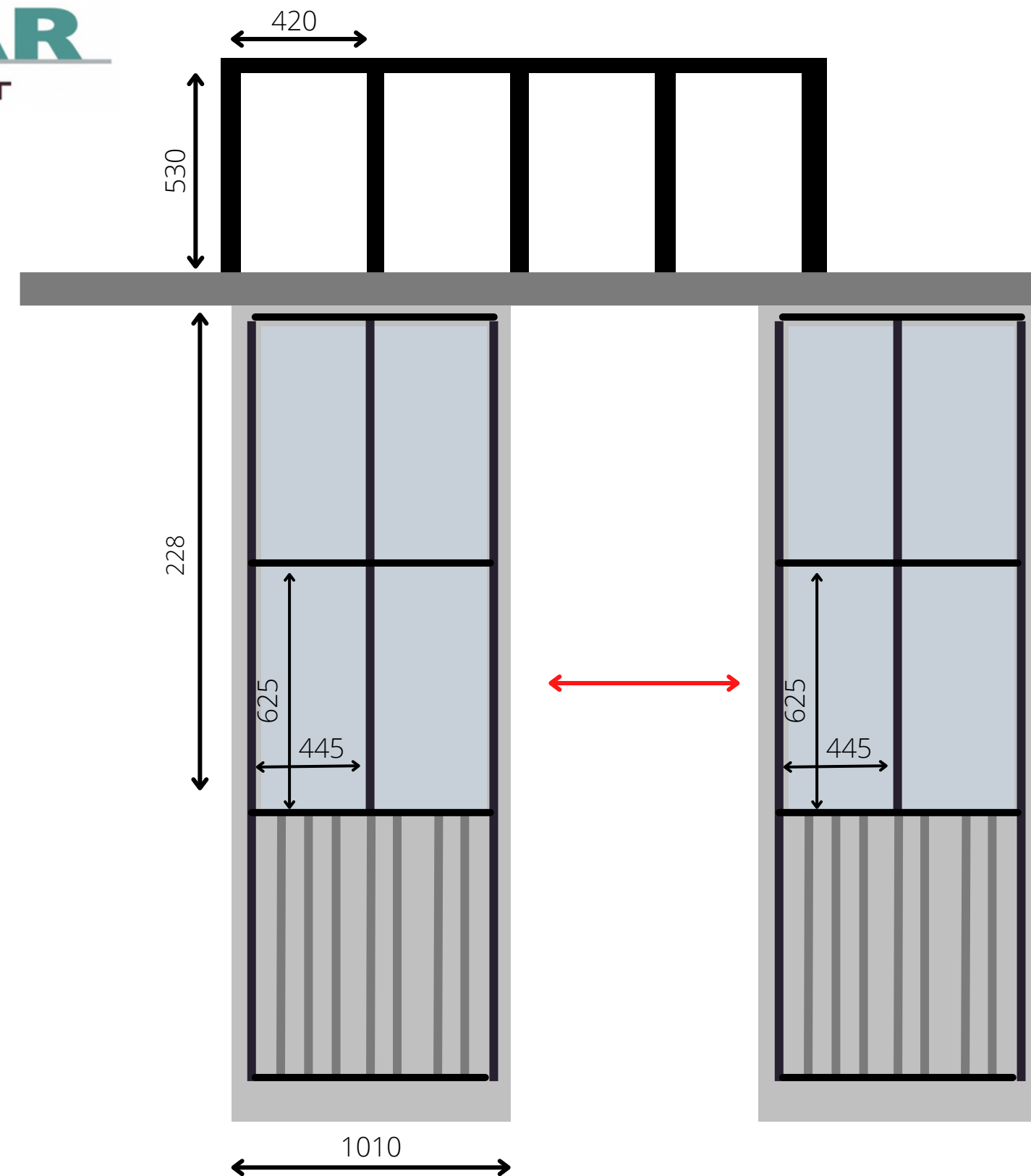
AFMETINGEN ZIJGEVEL MET DEUREN
